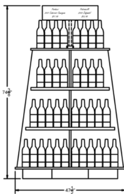
ELEVATION -C-
